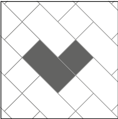
9 30x60 - 66,6% 20x40,4 - 66,6% 30x30 - 33,3% 20x20 - 33,3%
